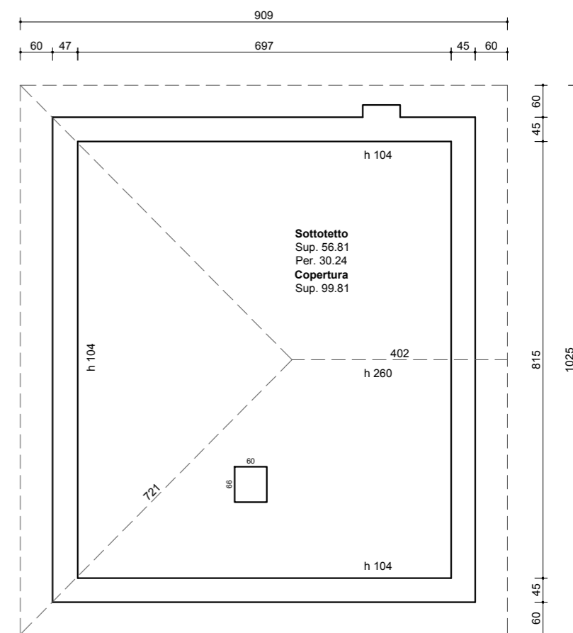
Piano sottotetto Scala 1/100
