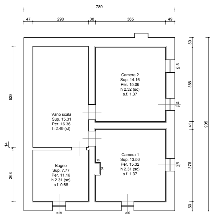
Piano secondo Scala 1/100
